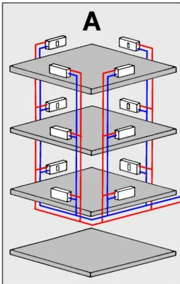
A DISTRIBUZIONE VERTICALE colonne montanti
