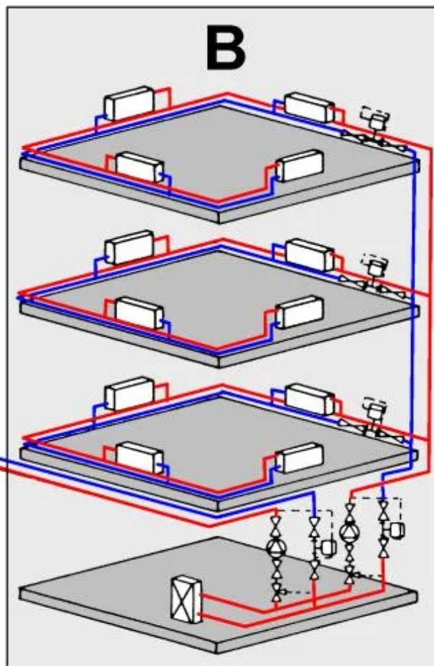
A DISTRIBUZIONE ORIZZONTALE tubazioni ad anello
